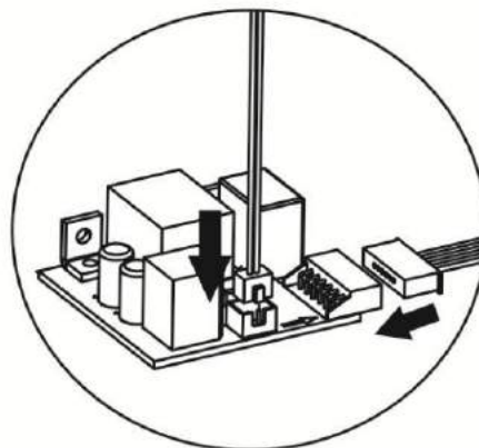
Коммуникационная плата
