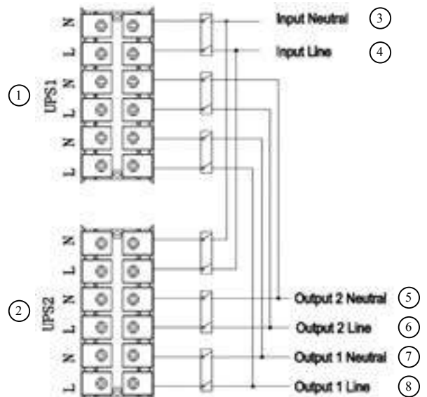
Рис. 10: Подключение кабеля питания
